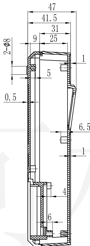
Section A-A
