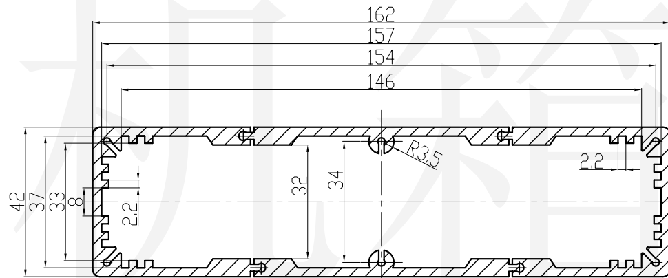
机箱壳体截面
