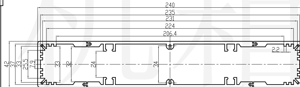
机箱壳体截面
